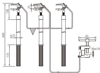
付属品: 収納袋、打込接地棒
