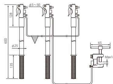
付属品: 収納袋、打込接地棒
